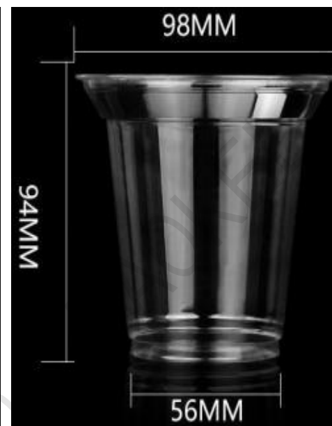
98mm-12oz 340ml
